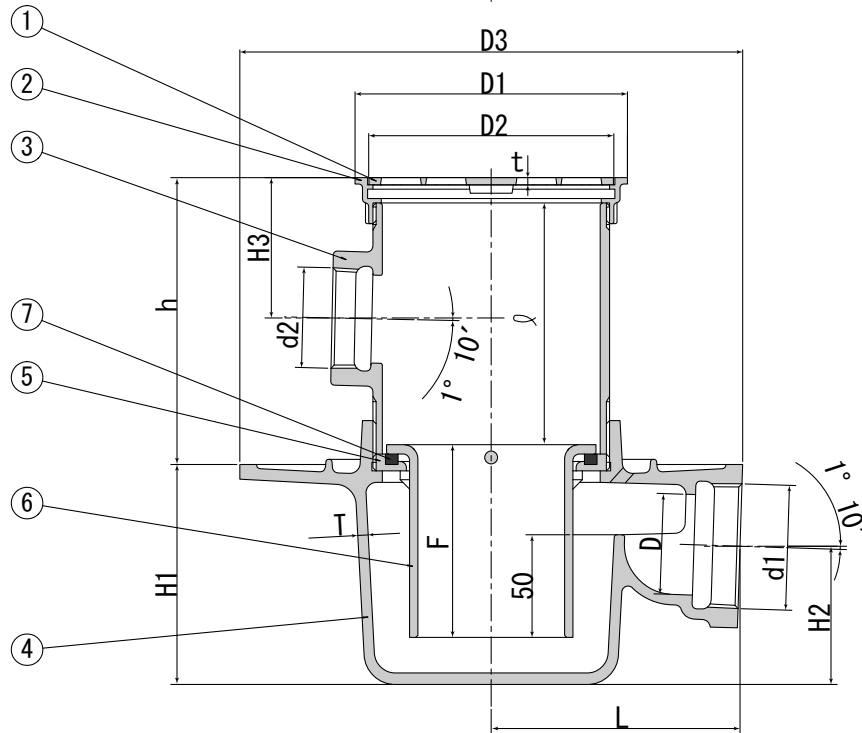
回転引き上げ バー付封水筒
