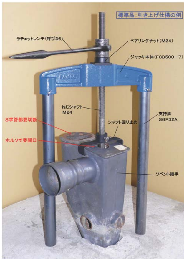
プルッシュジャッキを用いてソベント継手を引き抜く動画
