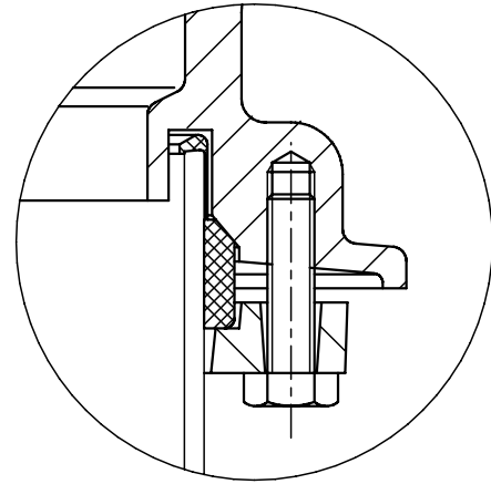
A部拡大詳細図
