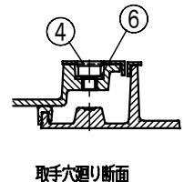
取手穴廻り断面
