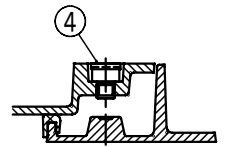
取手穴廻り断面
