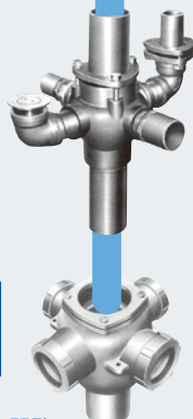
扁球体多口管継手
