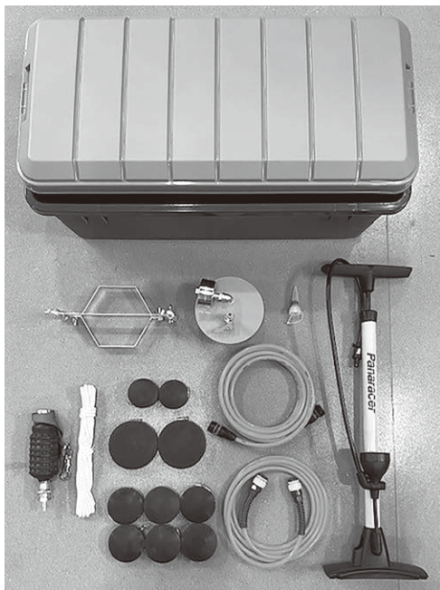
満空試験治具 標準セット (写真LTCS 100)
