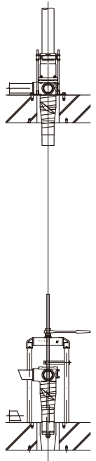
⑥ジャッキで下部継手を抜く
