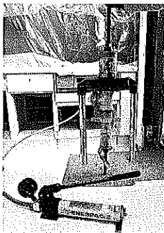
引き抜き完了後の「手動油圧ジャッキ」全体像騒音・震動・粉塵を出さずに引き抜き
