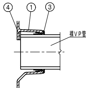
横枝管接続部詳細
