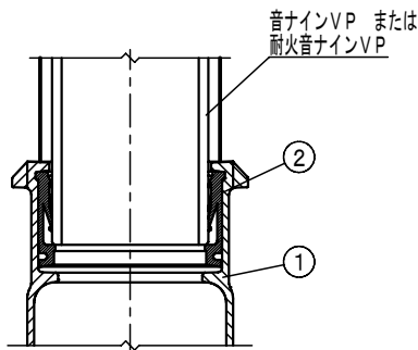
上部立て管接続部詳細
