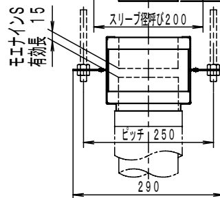
別紙E-X-Em-Bush施工手順書参照 E-X-Em-Bush接続部詳細
