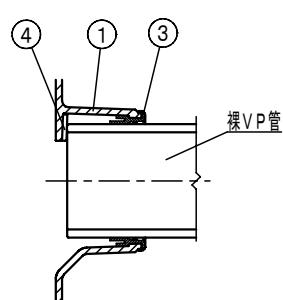
横枝管接続部詳細
