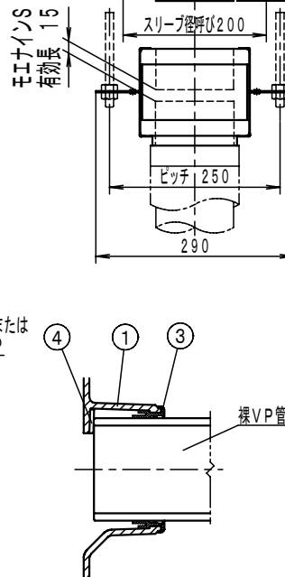
横枝管接続部詳細
