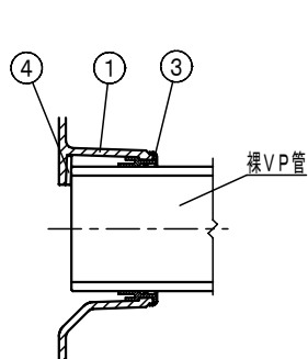
横枝管接続部詳細
