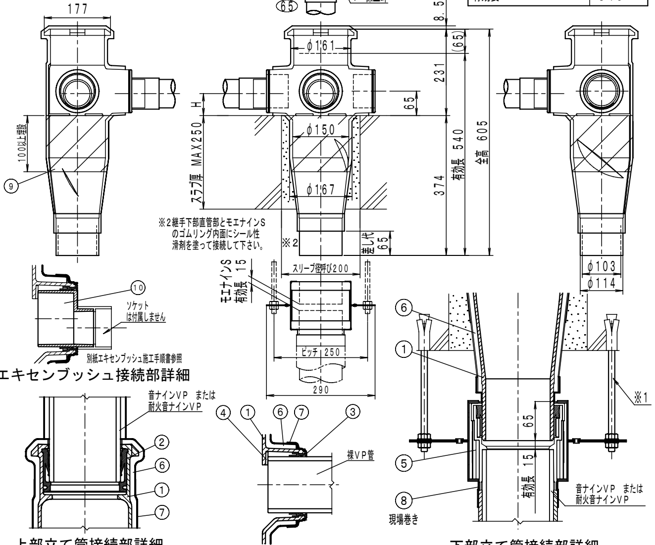
横枝管接続部詳細
