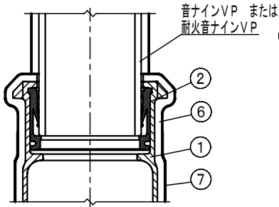
上部立て管接続部詳細
