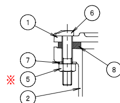
上部継手と下部継手 との接続部形状
