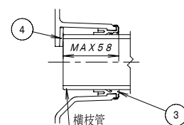
横枝管 横枝管接続部形状
