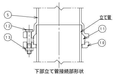
下部立て管接続部形状
