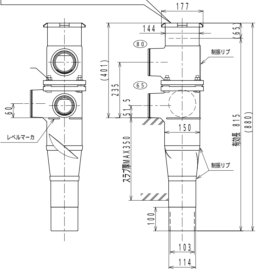
上部立て管接続部形状
