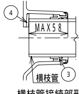
横枝管接続部形状
