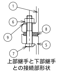
上部継手と下部継手との接続部形状
