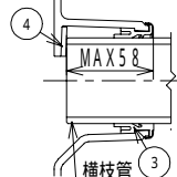
横枝管接続部形状
