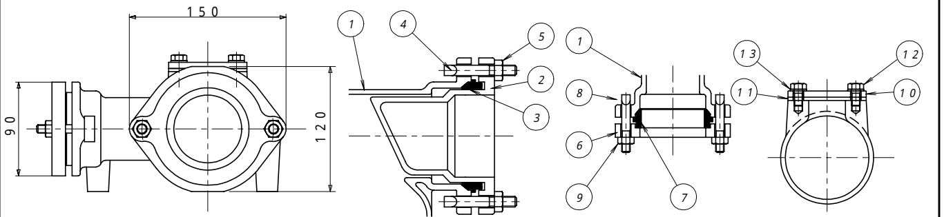
横枝管接続部形状
