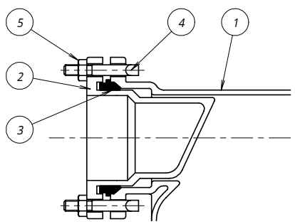
三角ふた装着部形状
