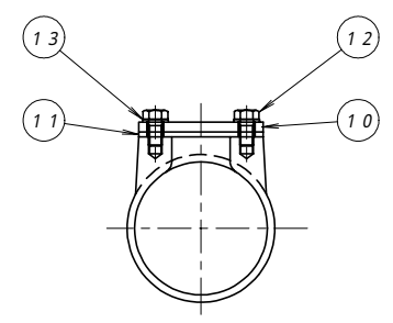
点検口ふた装着部形状
