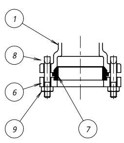
横枝管接続部形状
