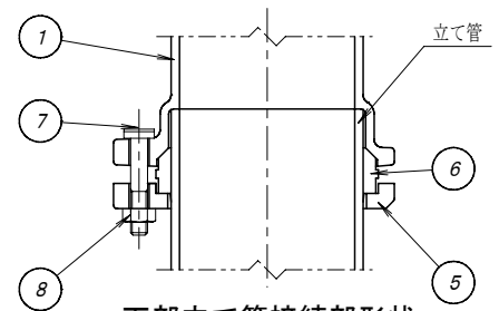
下部立て管接続部形状
