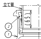
上部立て管接続部形状
