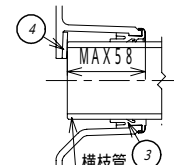
横枝管接続部形状
