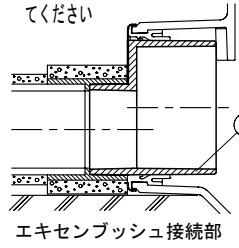
■部品図
