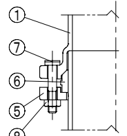
下部立て管接続部
