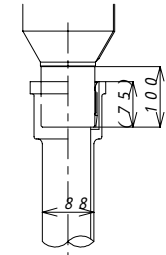
R-J排水用铸铁管 JSSA規格
