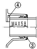
横枝管接続部
