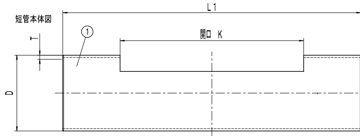
■寸法表
