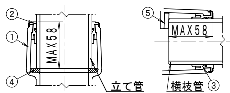
上部立て管接続部形状 横枝管接続部形状
