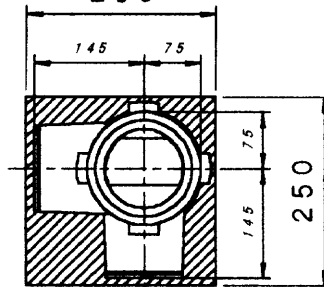
2方向(L)型 250
