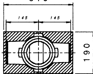
2方向(I)型 310
