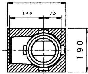
1方向型 250
